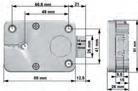
StraightBolt
