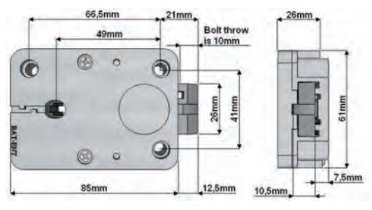
Motor SpringBolt
